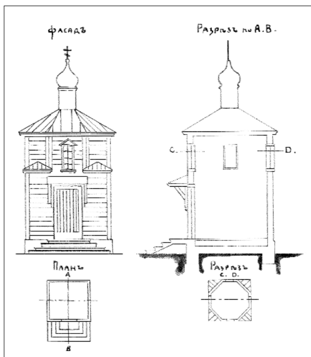
Часовня на кладбище в деревне Филатово. Чертеж из фондов ЦИАМ
